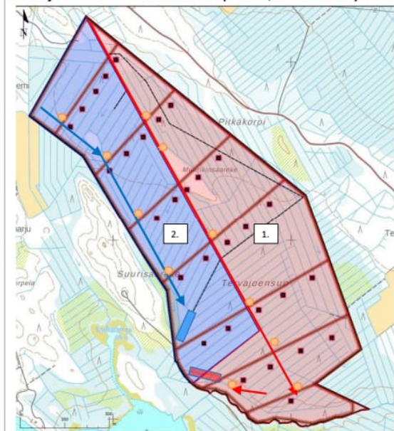
Kartta 13. Periaatepiirros aurinkovoimala-alueen valumavesien viivyttämistä. (Lähde: Envineer Oy)
